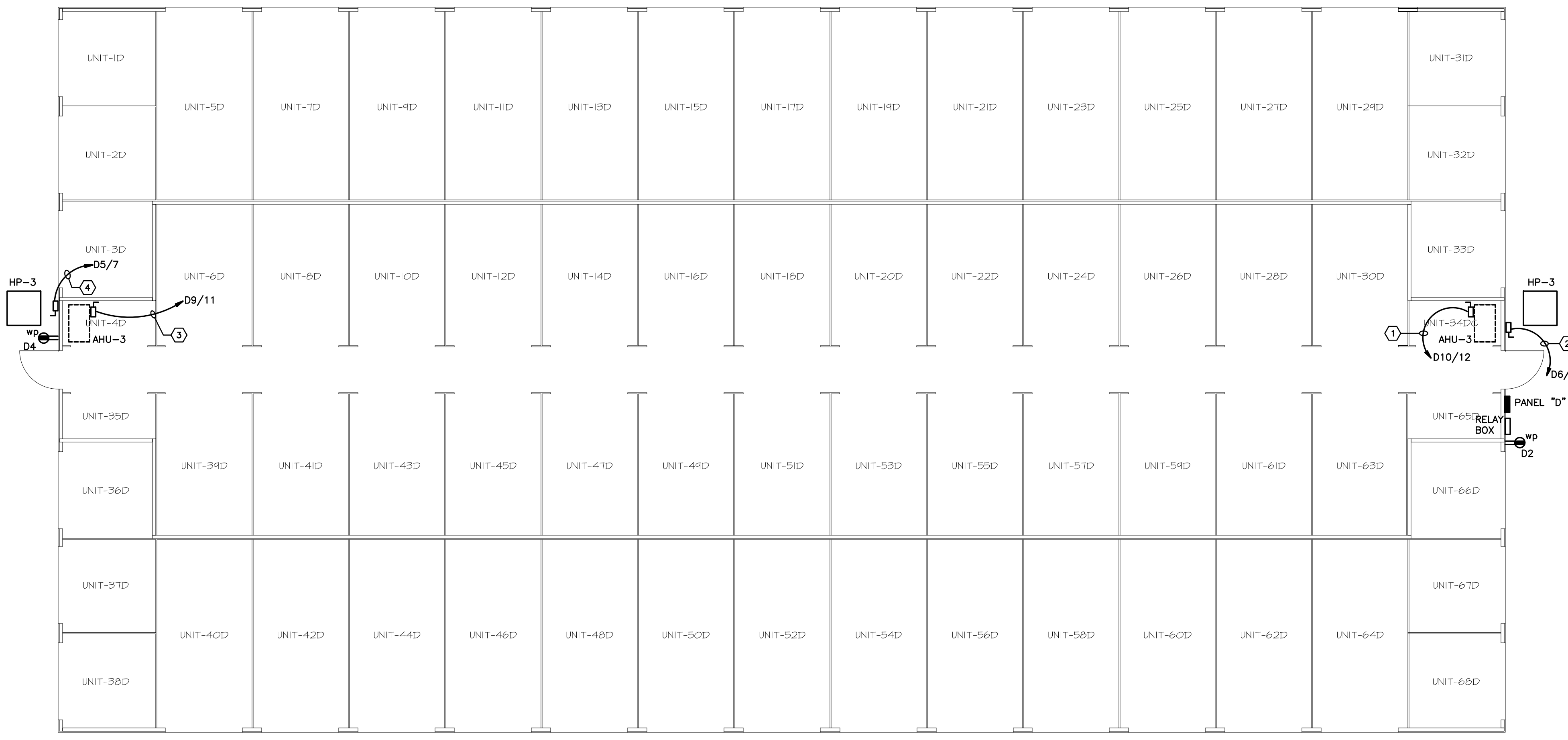
2 BLDG. "D" - POWER E2.4 SCALE: 1/8" = 1'-0"
